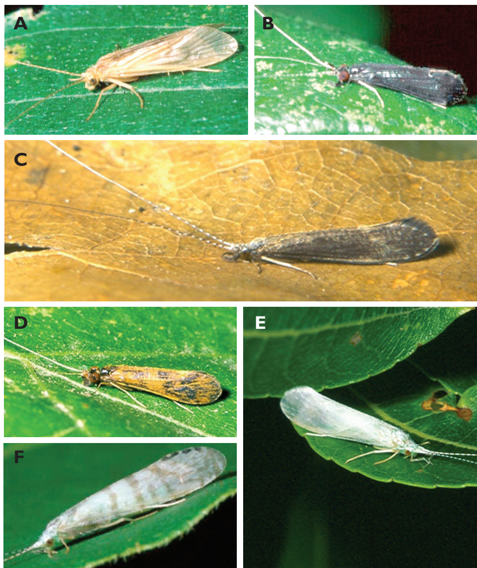
Figure 291. Adult specimens of A Potamyia flava (Hydropsychidae) B Mystacides sepulchralis (Leptoceridae) C Leptocerus americanus (Leptoceridae) D Mystacides interjecta (Leptoceridae) E Nectopsychidae candida (Leptoceridae) F Nectopsyche exquisita (Leptoceridae).
