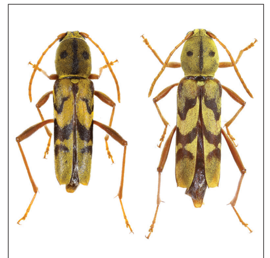
Xylotrechus tristisfacies S. Yang & W. Yang, sp. n.
